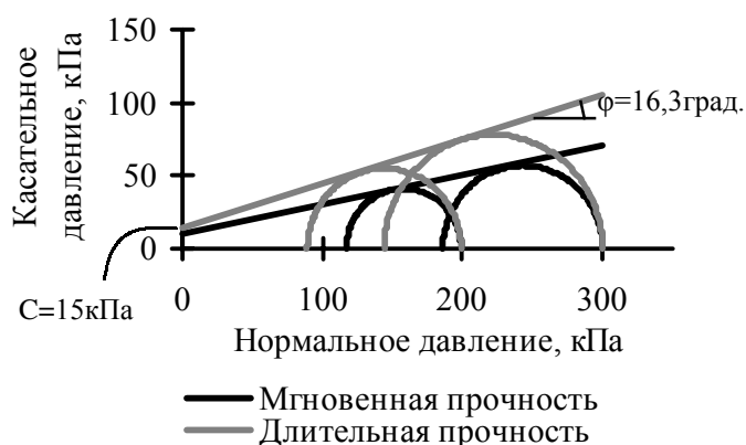
Графики испытаний на прочность образца с глубины - 3,0м от дна котлована
