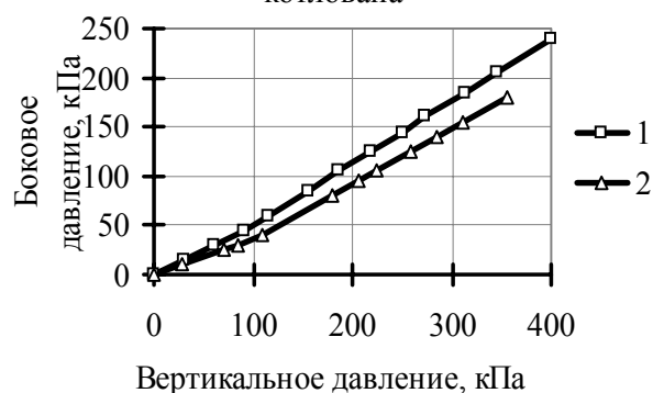
Паспорт компрессионных испытаний образца с глубины - 3,0м от дна котлована
