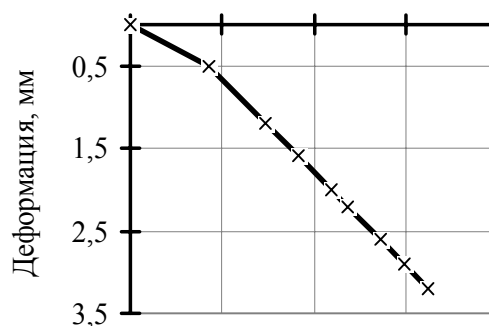
Рис. 2. Зависимость боковых напряжений от деформации
