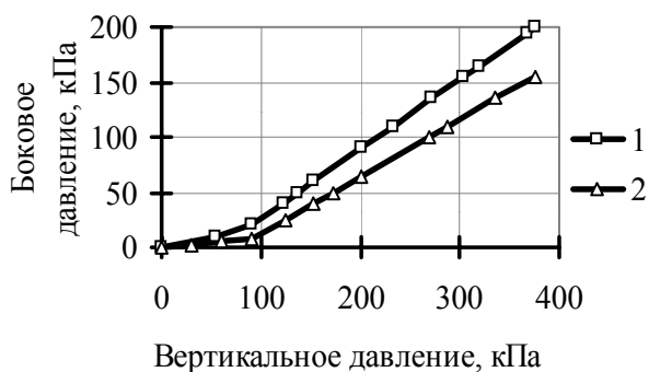
Паспорт компрессионных испытаний образца с глубины - 1,5м от дна котлована
