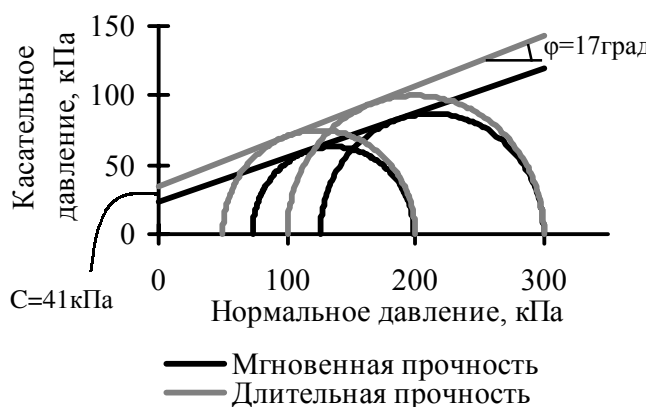
Графики испытаний на прочность образца с глубины - 1,5м от дна котлована
