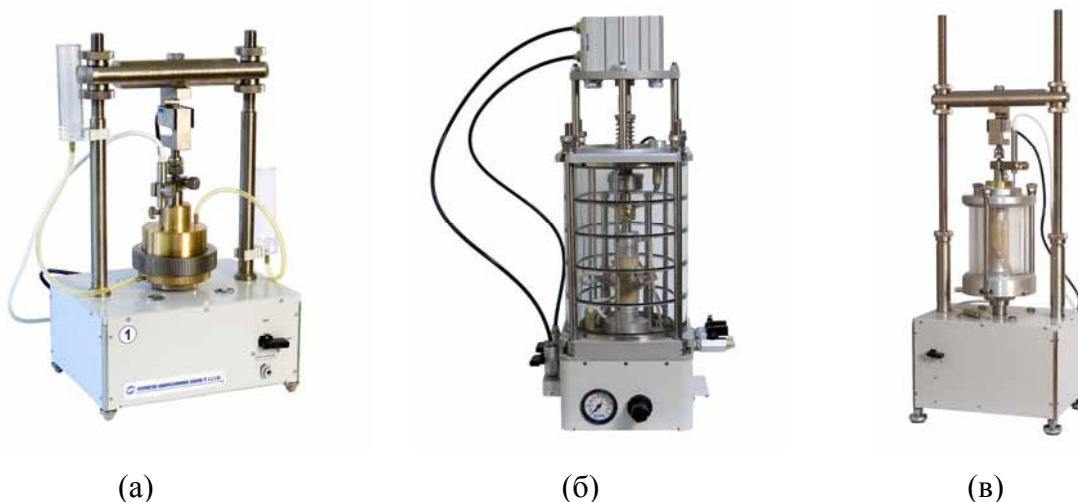
Рис. 1. Приборы для испытания образцов грунта, конструкции ООО «Геотек»: а – компрессионный прибор; б – прибор трехосного сжатия, тип А; в – прибор трехосного сжатия тип, Б
