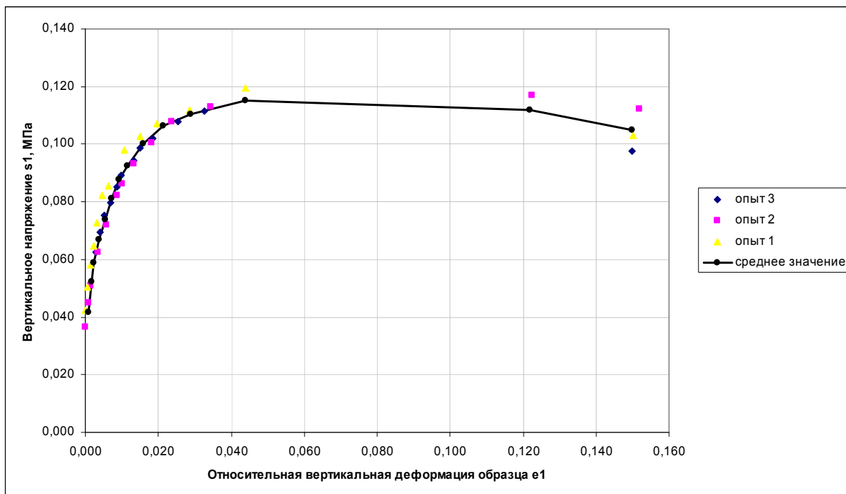
Рис. 7. Зависимость относительной вертикальной деформации от вертикального напряжения при постоянном боковом напряжении, равном 30 кПа штамповым, а это возможно только при резком уменьшении боковых напряжений. С этой целью были проведены испытания песка в стабилометре при боковом давлении в 30 кПа,
